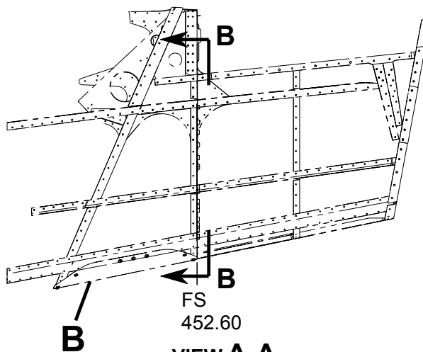
VIEW A-A
